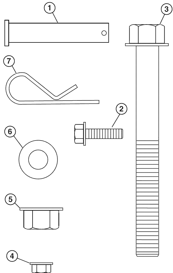
Figura 3 – Elementos de ferretería del kit de las ruedas – número de serie XXXXXX0612 y antes
