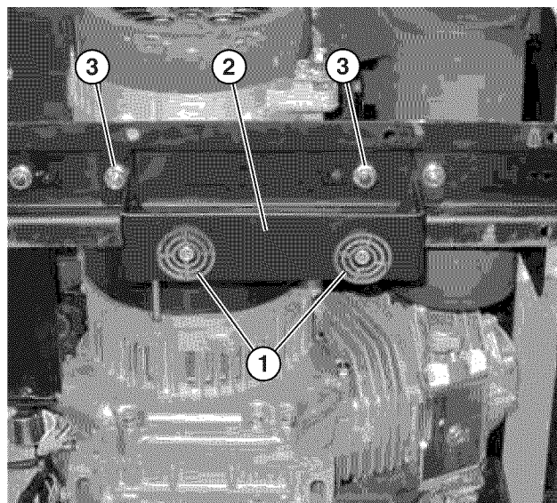
Figura 12 – Ensamble el pie de montaje al bastidor
