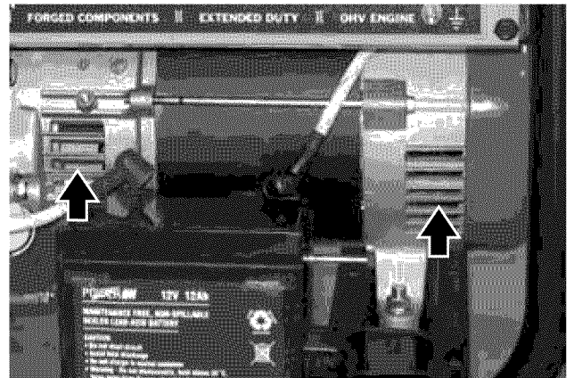
Figura 47 – Entrada de aire de refrigeración y orificio de escape del alternador
