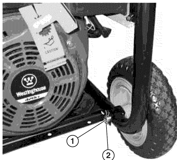
Figura 13 – Ensamble las ruedas al bastidor
