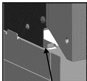
El panel del lado del fogón se apoya detrás de la pestaña vertical
