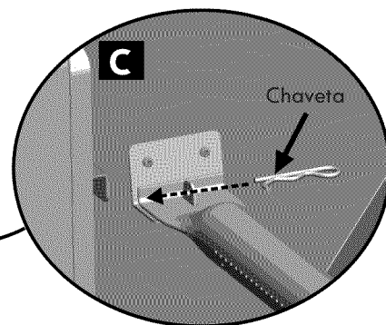
Chaveta Cant. 1
