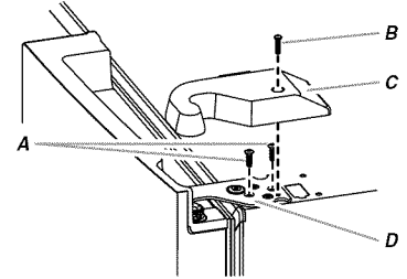
A. Tornillos internos de cabeza hexagonal de 3/16"
