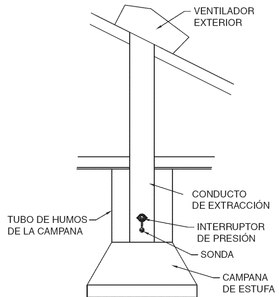
INSTALACIÓN TÍPICA CON VENTILADOR EXTERIOR
