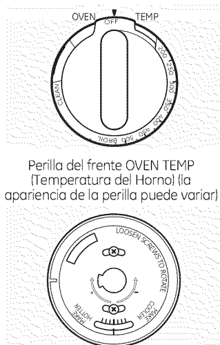
Perilla de la parte trasera OVEN TEMP (Temperatura del Horno) (la apariencia de la perilla puede variar)
