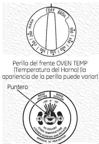
Perilla de la parte trasera OVEN TEMP (Temperatura del Horno) (la apariencia de la perilla puede variar)
