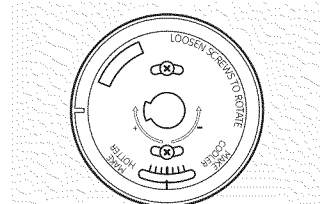
Perilla de la parte trasera OVEN TEMP (Temperatura del Horno) (la apariencia de la perilla puede variar)
