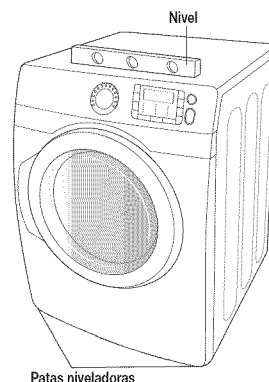
Patas niveladoras
