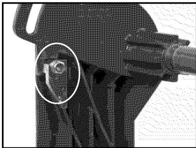
(D) Move Cutting Head Stop to down position.
