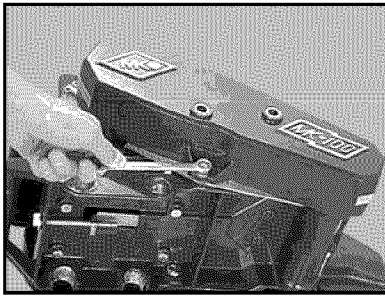
(D) Remove Belt Guard bottom bolt.
