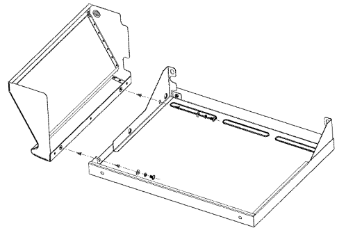
Tornillos de M4x10 Cant.: 1
