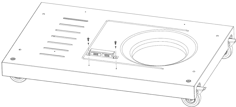
Tornillos de M4x10 Cant.: 2 us
