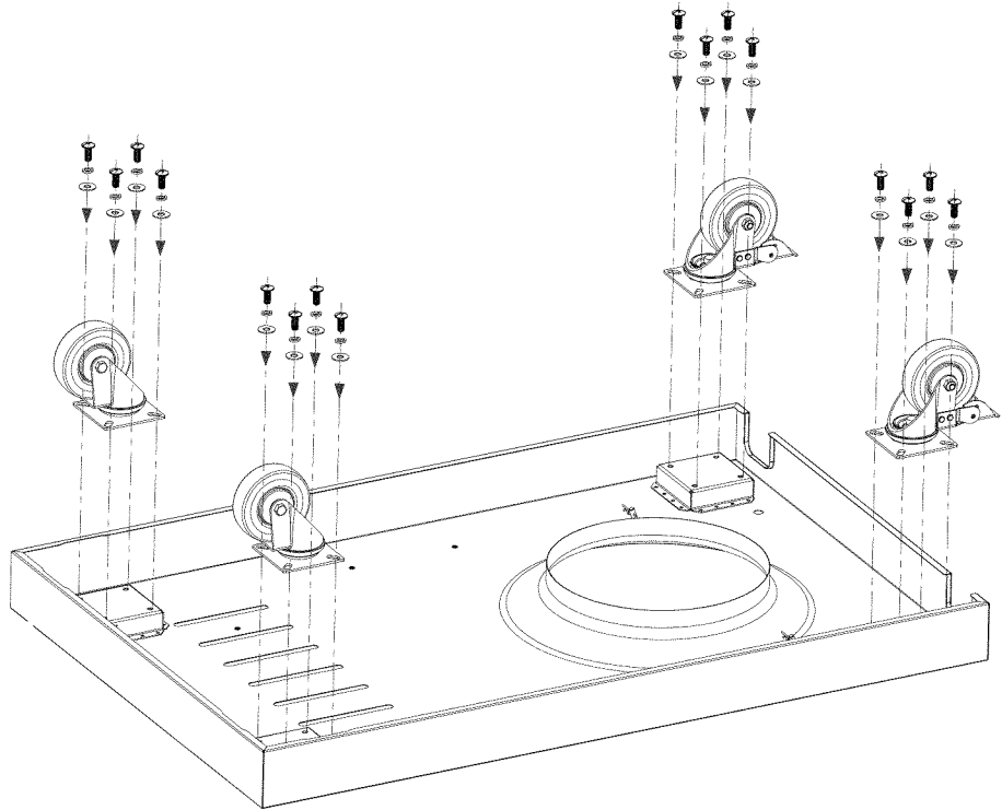
Tornillos de M4x15 Cant.: 16 us
