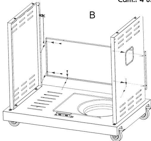
Arandelas de seguridad M6 Cant.: 4 us
