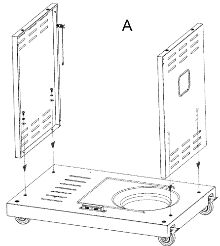
Arandelas de firba M6 (Dia 16) Cant.: 4 us
