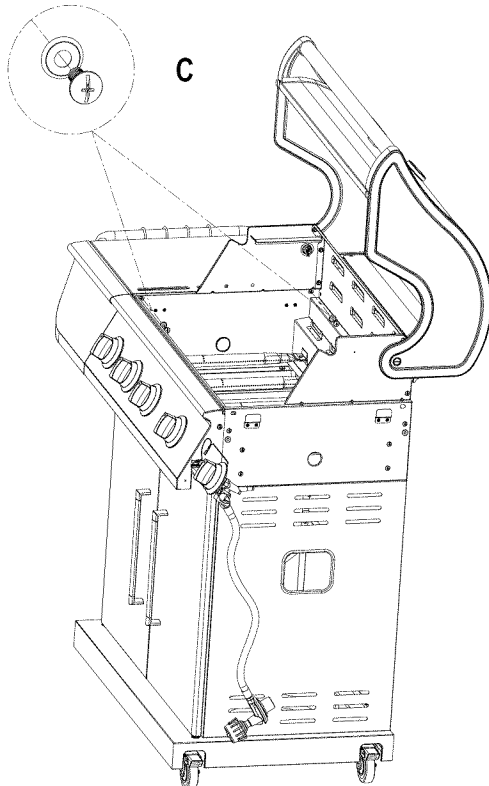
Arandelas de compresión de M6 Cant.: 2 us
