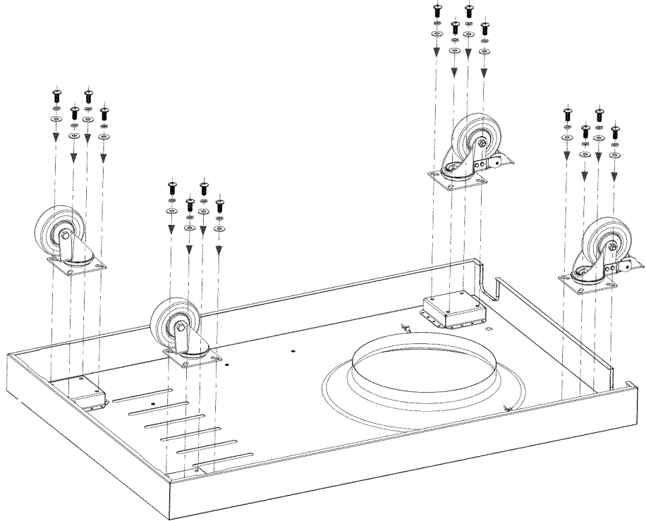
Tornillos de M6x15 Cant.: 16 us
