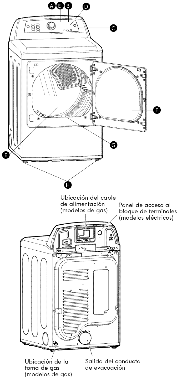
Parte posterior de la secadora
