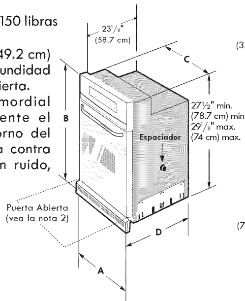
Figura 1- MODELOS CON UN SOLO HORNO (Modelos de horno doble vea la Figura 2)
