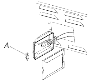
A. Abrazadera
