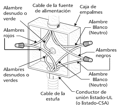
Figura 6 - Sistema eléctrico de 4 alambres (ejemplo caja de empalmes)
