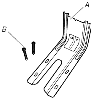
A. Bride antibasculement B. Vis de montage n° 12 x 1 5/8"
