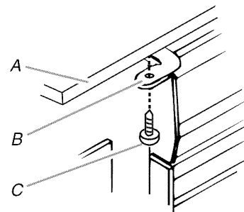
A. Mostrador B. Soporte de retención (provisto en el juego de conversión) C. Tornillo de montaje (provisto en el juego de conversión)
