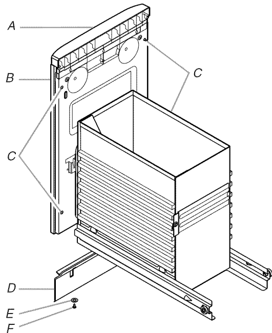
A. Poignée B. Panneau personnalisé C. Emplacements des vis du panneau D. Garde-pieds E. Rondelle F. Vis de montage du garde-pieds
