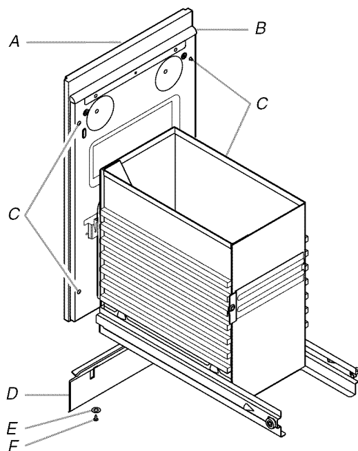
A. Panel personalizado B. Relleno de cuarto bocel de 15" (38,1 cm) x \frac{1}{2} " (13 mm) C. Ubicaciones de los tornillos del panel D. Guardapiés E. Arandela F. Tornillo de montaje para guardapiés
