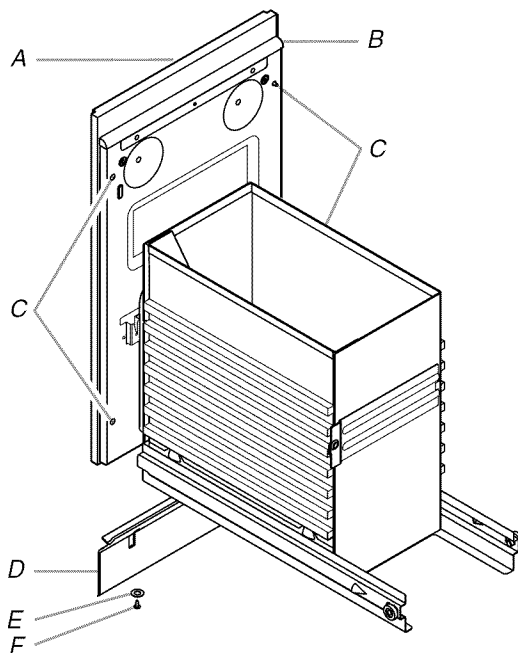
A. Panneau personnalisé B. Quart-de-rond de 15" (38,1 cm) x 1/2" (13 mm) C. Emplacements des vis du panneau D. Garde-pieds E. Rondelle F. Vis de montage du garde-pieds
