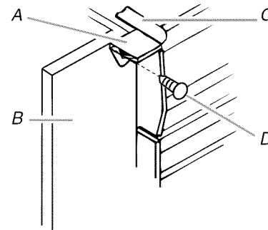
A. Agrafe de montage (fournie dans la trousse de conversion)
