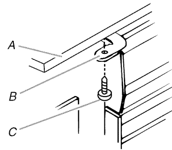
B. Bride de retenue (fournie dans la trousse de conversion)
