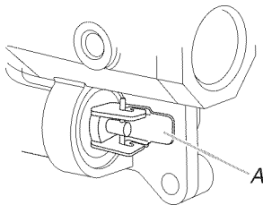
A. Robinet d'arrêt du détendeur montré en position "ON" (ouvert)
