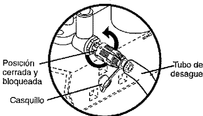
Válvula de desague del aceite
