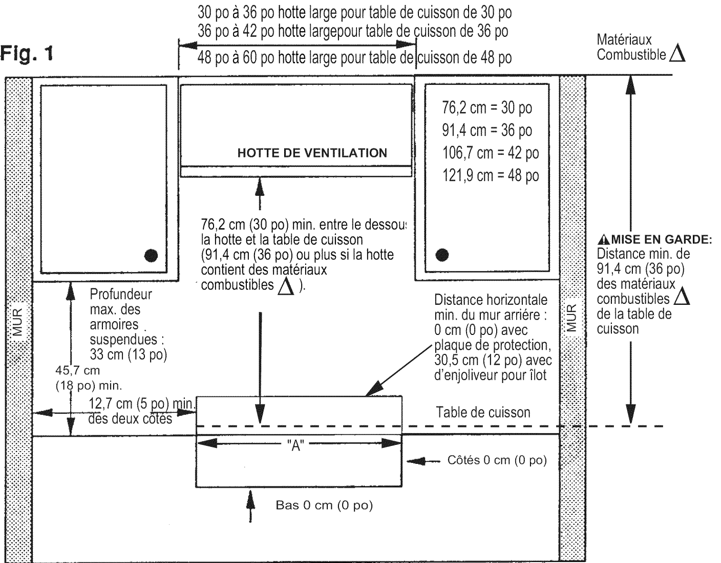
Figure 1 : Dégagements
