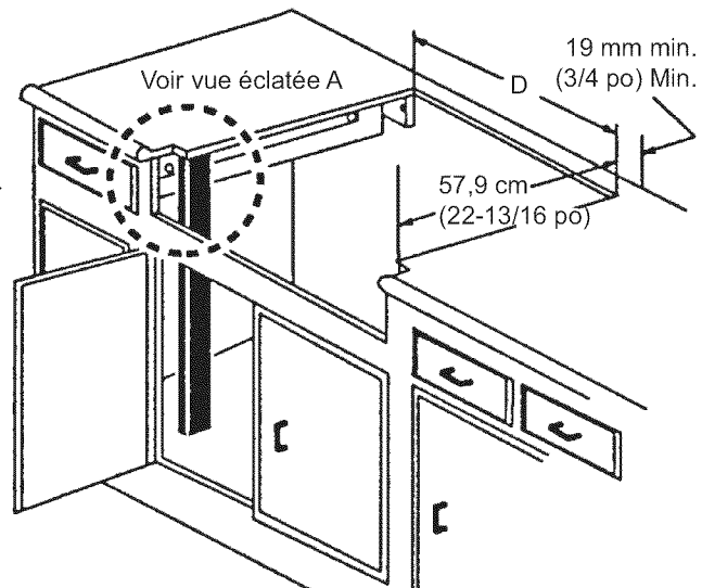
Figure 4 : Installation en îlot (sans rebord de plan de travail)
