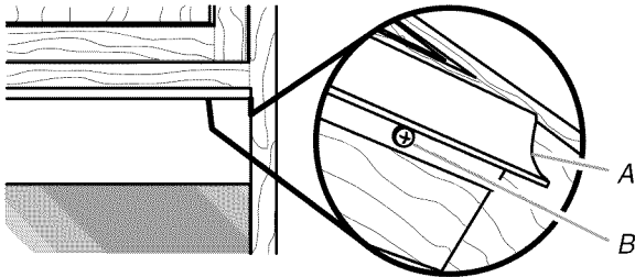
A. Moldura de la rejilla superior B. Tornillo de cabeza hexagonal ranurada
