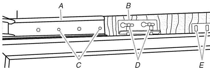
A. Charnière supérieure B. Support supérieur de panneau C. Trous pour les vis D. Tiges de réglage de porte E. Modèles de 36" uniquement - Trous pour les vis
