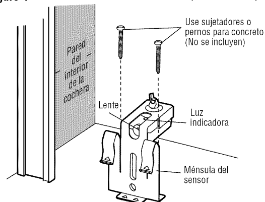
Figure 4 INSTALACIÓN EN EL PISO (LADO DERECHO)
