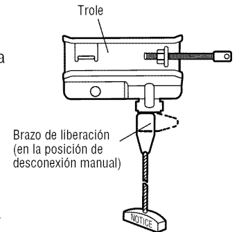
Posición con el seguro (desconexión manual)
