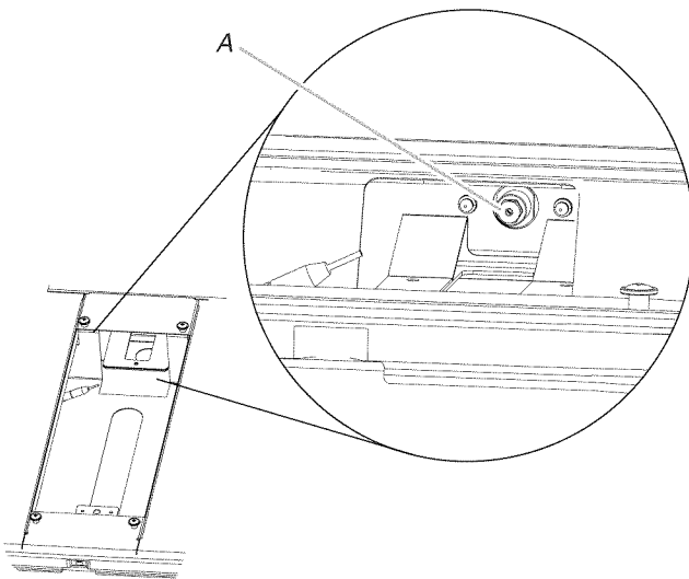
A. Gas orifice spud
