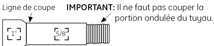
Installation avec un raccord en té d'égout Figure II
