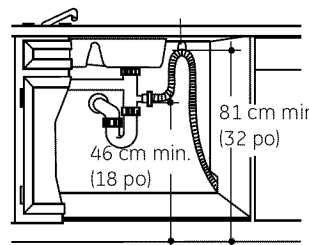
Installation avec un raccord en té d'égout Figure II
