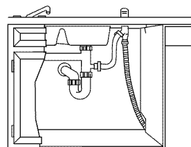
Installation avec un raccord en té d'égout Figure HH
