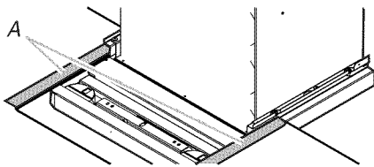
A. L-bracket
