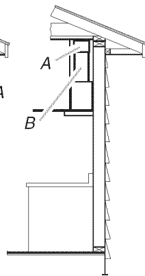
A. Déflecteur B. Conduit dia. 8" (20,3 cm)
