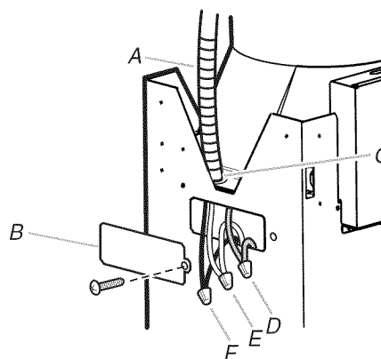
A. Conduit de 1/2" B. Couvercle de la boîte de connexion C. Serre-câble (homologation UL ou CSA) D. Conducteur vert (ou nu) connecté au conducteur jaune/verte E. Conducteurs blancs F. Conducteurs noirs
