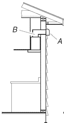
A. Bouche de décharge murale B. Conduit dia. 8" (20,3 cm)
