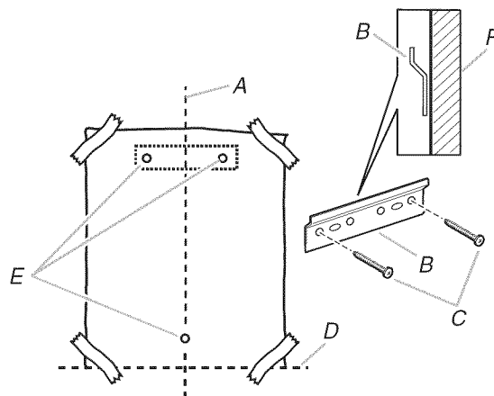
A. Axe central B. Bride de support inférieure C. Vis de 5 x 35 mm D. Ligne de référence - hauteur de montage E. Emplacements des organes de fixation F. Mur
