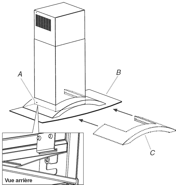
A. Vis du cache-conduit (section inférieure) B. Vitre C. Garniture esthétique
