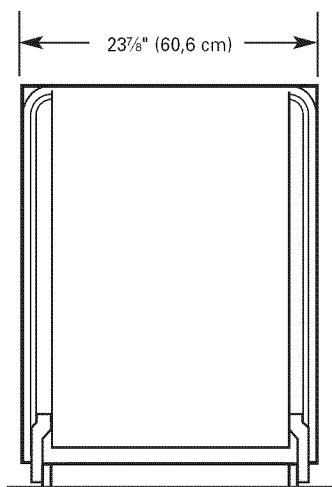
VUE ARRIÈRE
