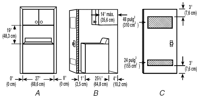
A. Vista frontal B. Vista lateral C. Puerta del clóset con orificios de ventilación
