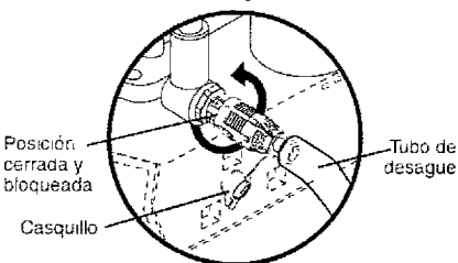
Válvula de desagüe del aceite
