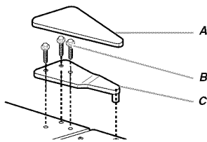
A. Plaque de charnière supérieure B. Vis de charnière à tête hexagonale de 3/16" C. Charnière supérieure
