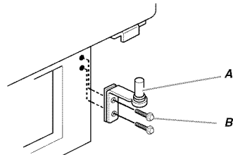
A. Charnière inférieure B. Vis de charnière à tête hexagonale de 3/16"
