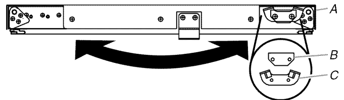
A. Bas de la porte du réfrigérateur B. Cale d'espacement de la butée de porte C. Butée de porte
