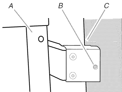
A. Partie avant de la porte B. Trou de vis de la bride latérale pour la fixation du placard C. Avant du placard
