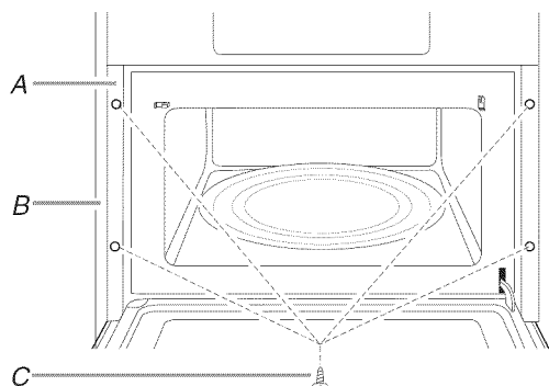
A. Encadrement de façade de la porte du four à micro-ondes B. Placard C. Vis T-10 de 1" (4)
