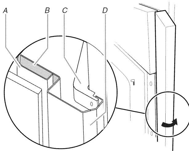
A. Encadrement faisant face à la porte B. Partie tabulaire (grisée) du panneau de garniture latérale C. Bride latérale D. Panneau de garniture latérale installé
