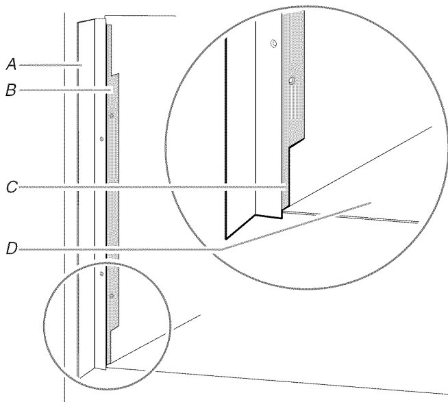
A. Support de montage B. Bord mixte (grissé) C. Partie plus étroite D. Plancher de l'ouverture
