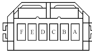
MÓDULO DE SEGURIDAD ES VISTO DESDE LADO DE CONECTANDO
