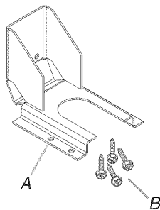
A. Bride antibasculément B. 4 vis à tête Phillips n° 8-18 x 1"
