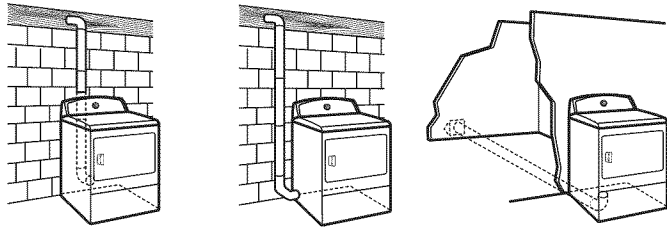
A. Instalación estándar con ventilación en la parte posterior B. Instalación de ventilación lateral a la izquierda o a la derecha C. Instalación con ventilación por la parte inferior
