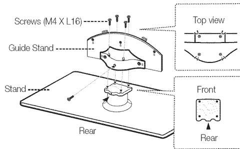
Guide Stand (1EA)
