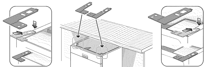
Montaje superior
