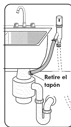
A la conexión de drenaje para lavadora de platos de un triturador de desechos a través de un espacio de aire.
