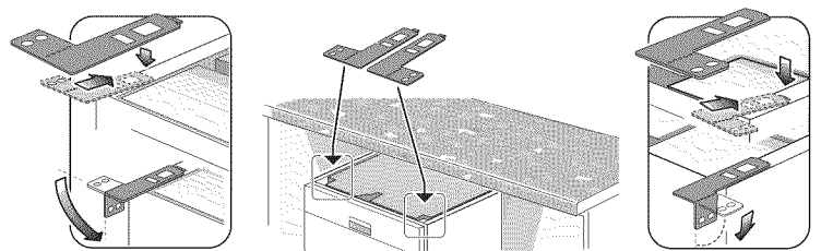
Montaje lateral
