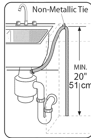
Directamente a la conexión de drenaje para lavadora de platos de un triturador de desechos.
