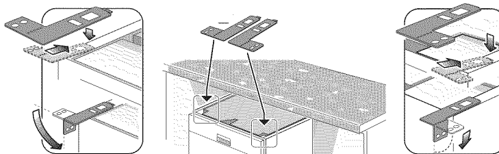
Méthode de fixation latérale
