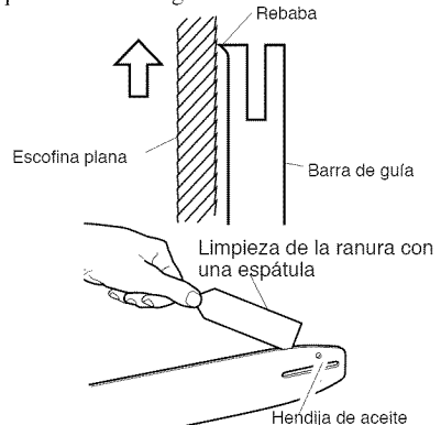
Figura 21 - Mantenimiento de la barra de guía
