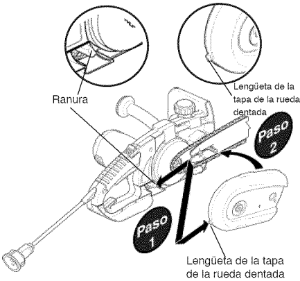
Figure 7- Instalación de la tapa de la rueda dentada
