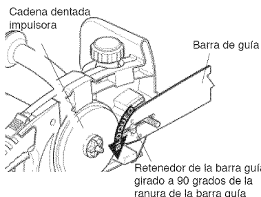
Figura 3 - Bloqueo del retenedor de la barra guía
