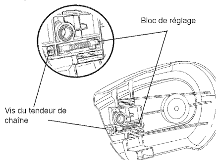
Figure 5 - Emplacement de la vis de tendeur de chaîne et du bloc de réglage
